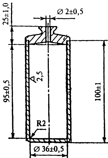
Рисунок 3 — Пикнометр
