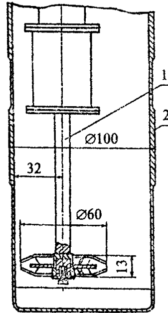
1 - лопастное устройство; 2 - стакан Рисунок 1 - Смеситель лопастной
