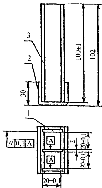
Рисунок 5 — Форма размером 20x20x100 мм
