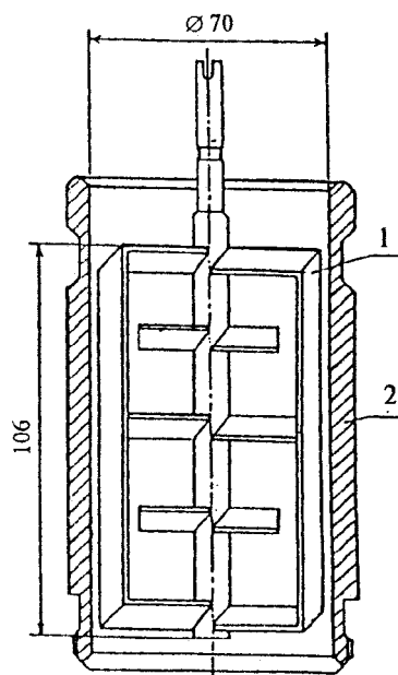
Рисунок 4 — Схема измерительного узла консисометра
